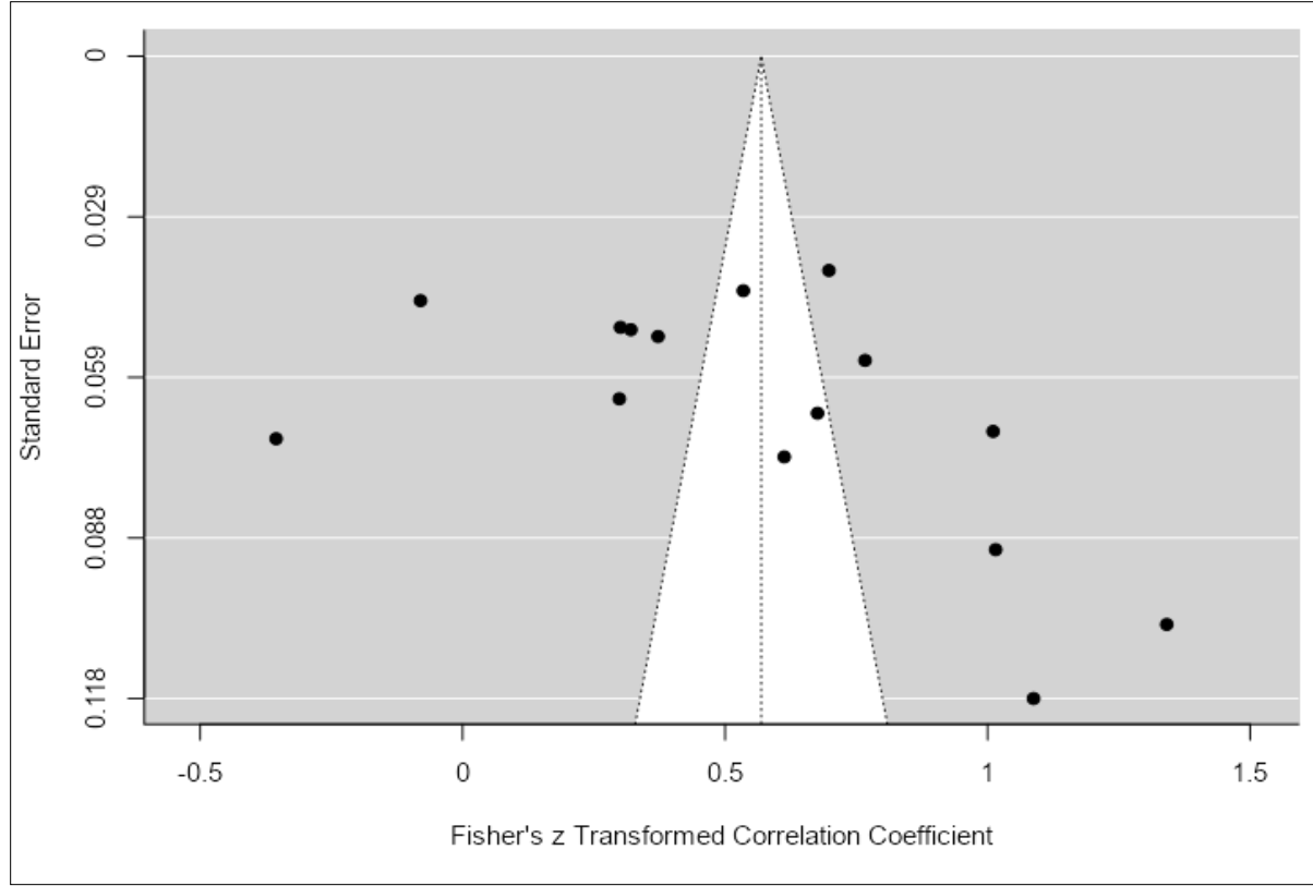
Şekil 1. Huni Grafiği
